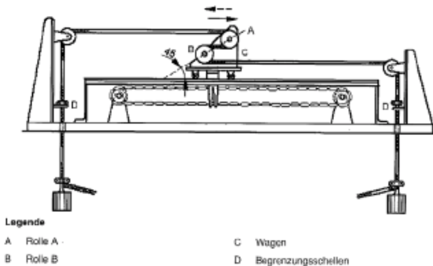
Bild 4 - Biegegerät
